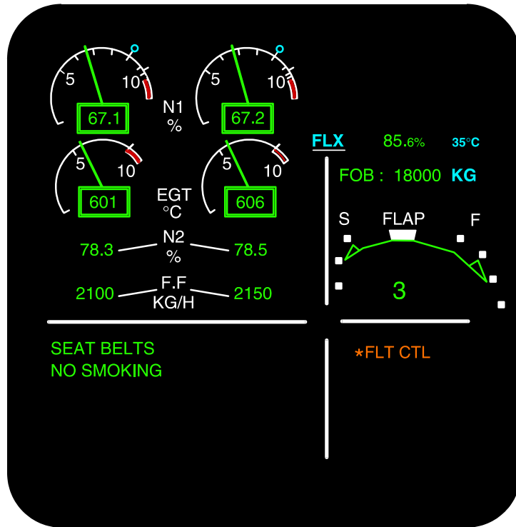
Upper display
